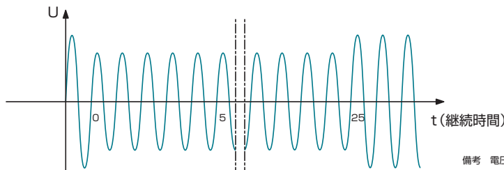
電圧ディップ例-70%電圧ディップ正弦波グラフ
