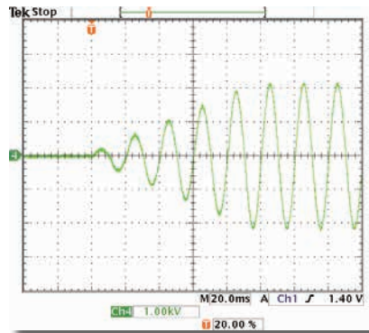
▲ライズタイム制御波形例
