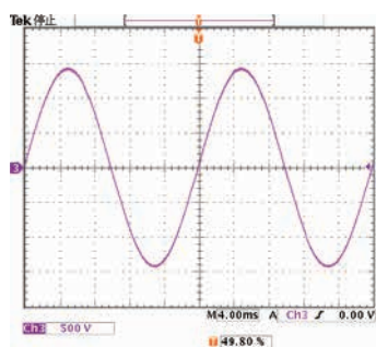
▲ TOS5200 の AC 出力波形
