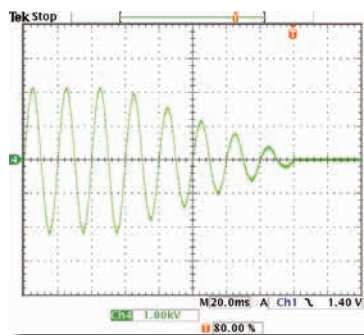
▲フォールタイム制御波形例
