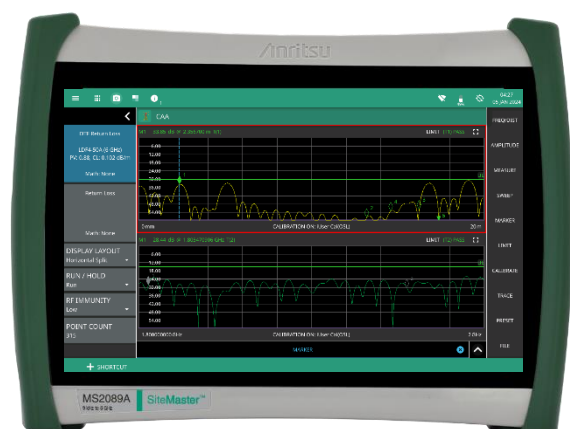
MS2085A/MS2089A ケーブル・アンテナアナライザ 画面
