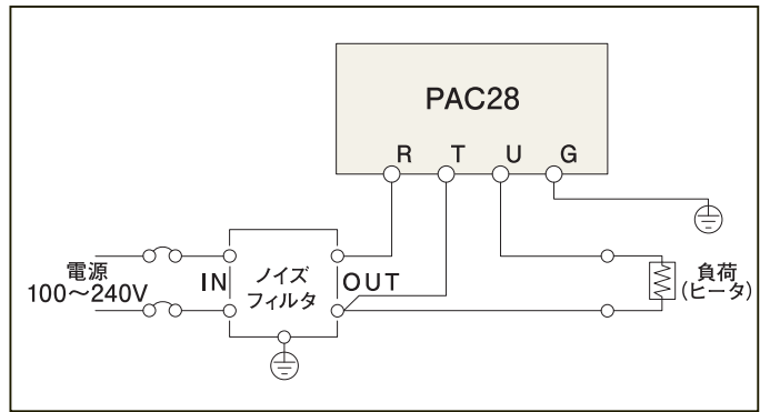
ノイズフィルタはPAC28と同一の金属板の上に設置し、接地を必ずとってください。 ノイズフィルタとPAC28間の配線はできる限り短くしてください。
