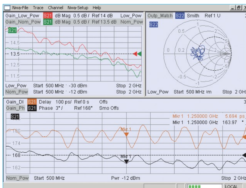
Multitrace display
