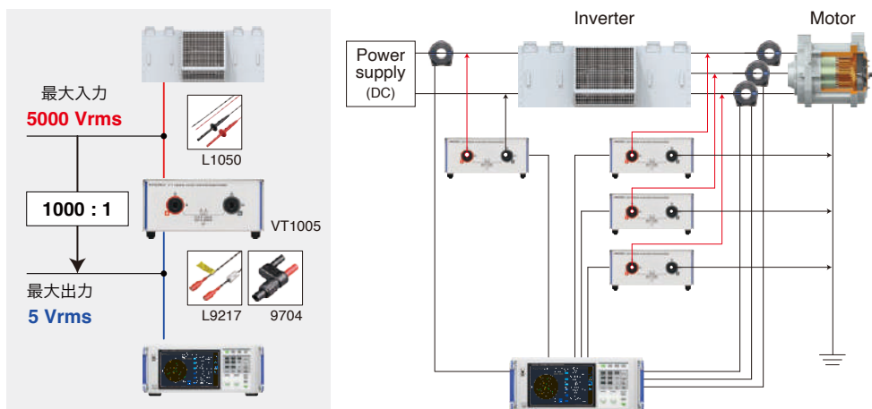
AC/DC ハイボルテージディバイダ VT1005
