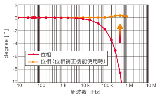
AC/DC カレントボックス PW9100A の位相特性補正例 (代表値)
