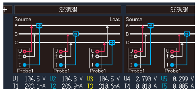
結線ミスを防ぐ結線確認機能
