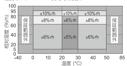
湿度センサ Z2000 使用時精度表
