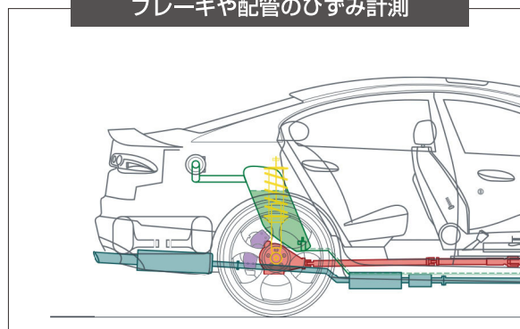
ブレーキや配管のひずみ計測
