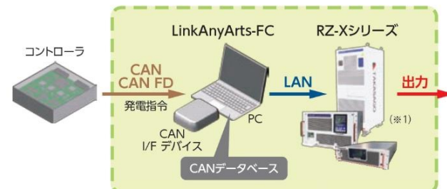
リアルタイムエミュレーションモードの構成
