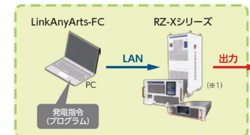
プログラムエミュレーションモードの構成
