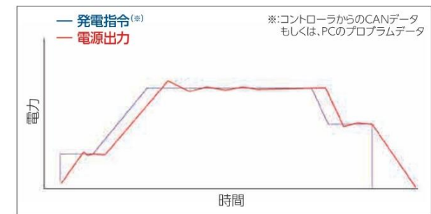
電源の出力波形の生成イメージ
