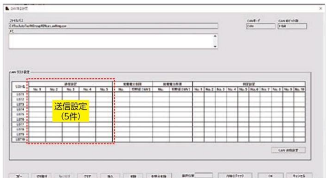
例: CAN項目設定画面* パターン編集で設定できるCAN送信設定・CAN判定設定・CAN充放電電力制限値の組み合わせを、プリセットとして10件分事前作成することができます。
