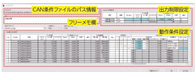
例: CANデータベースの登録設定画面* BMU連動で使用するCAN出力制限、CAN動作条件が設定できます。
