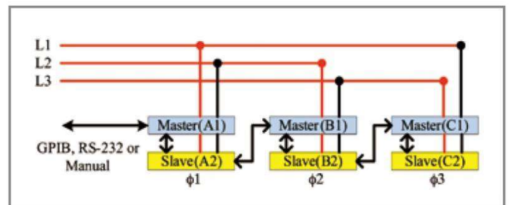
図 12: 並列三相 デルタΔ結線
