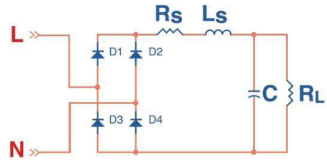
図2：代表的な整流回路
