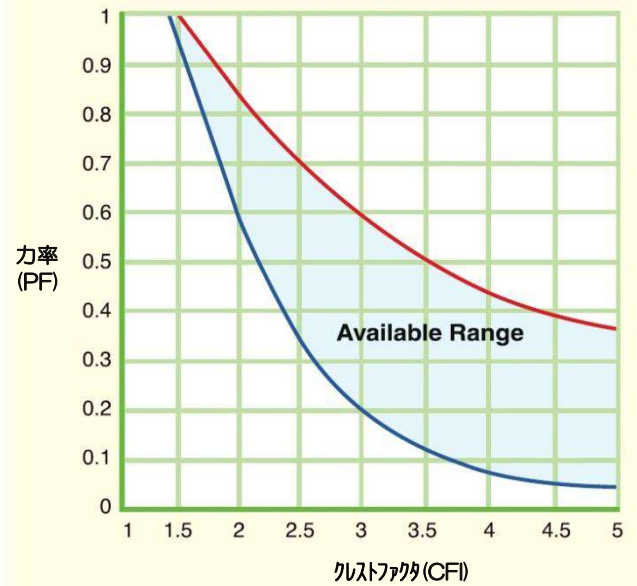
図1: クレストファクタ vs. 力率 (PF) 制御範囲
