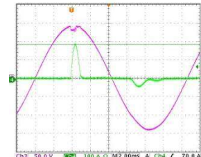
図6: 突入電流モード
