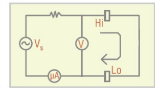
回路短絡時： C_m \gg C_x
