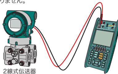
2線式伝送器
