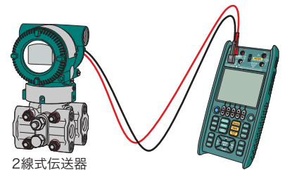
2線式伝送器
