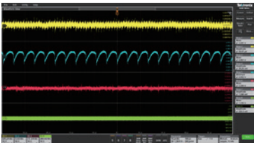
パワー・インテグリティ。パワーレール・プローブとオシロスコプの低ノイズ性能により、パワーレールの評価、解析を支援
