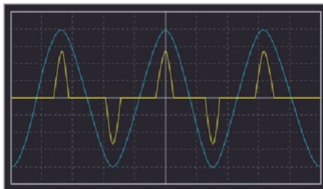
CFEモード動作波形 (CF=3)
