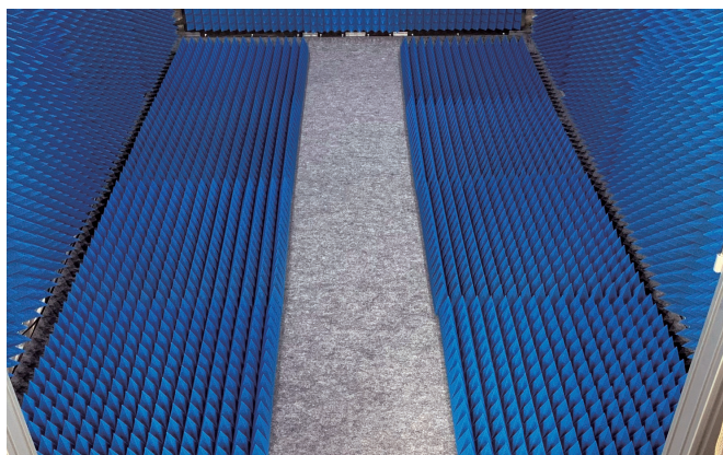
床面電波吸収体を部分的に取り外した状態
