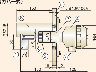
NL-15BY (保護カバー式)
