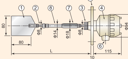
NL-8BA (振れ止めラバー型)
