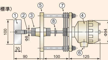
NL-8BHA (軸長調整式)
