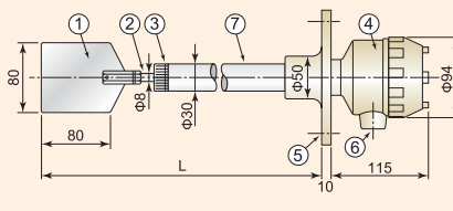
NL-8BS (スライドフランジによりL寸法調整可能)
