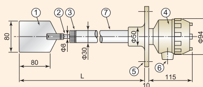
保護管延長式 NNL-8BS (安息角が大きい、タンク壁への付着が大きい場合等に、垂直取付・水平取付・斜め取付も可能)
