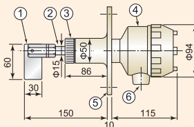
耐荷重式 NNL-15B (耐荷重式サイロ下限用レベルスイッチ)
