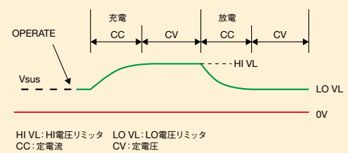
バッテリー充電波形
