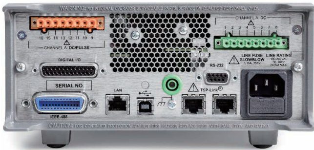
2601B-PULSE型の後部パネル
