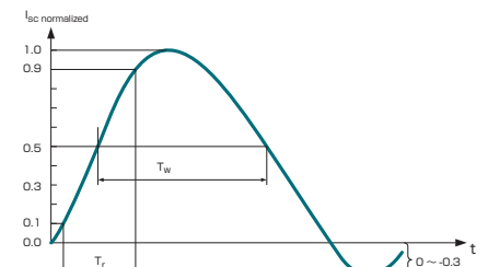
電流波形
