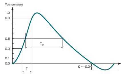
電圧波形
