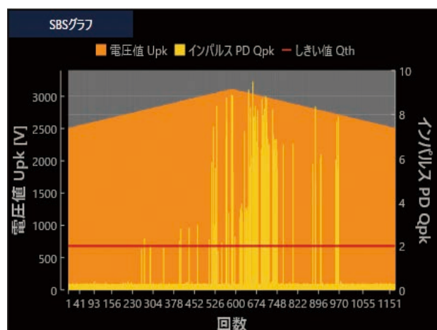
SBS 解析グラフ
