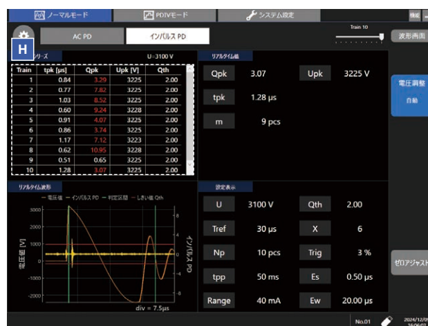
インパルス PD ノーマルモード測定
