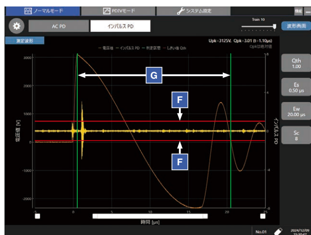
部分放電検出のしきい値と判定区間を設定
