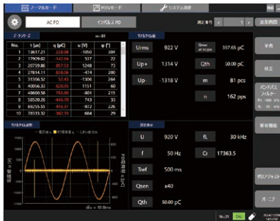
AC PD ノーマルモード測定
