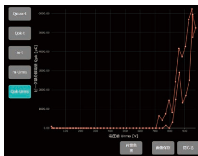
Qpk Urms 解析グラフ
