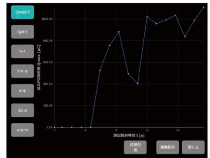
Qmax-t 解析グラフ
