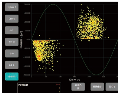
q-Φ -m 解析グラフ
