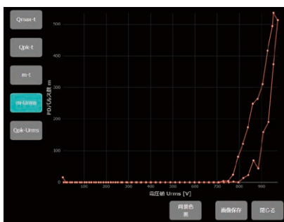
m-Urms 解析グラフ
