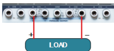
直列接続 (電圧2倍)
