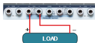
並列接続 (電流2倍)
