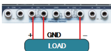
直列接続 (+/-出力)
