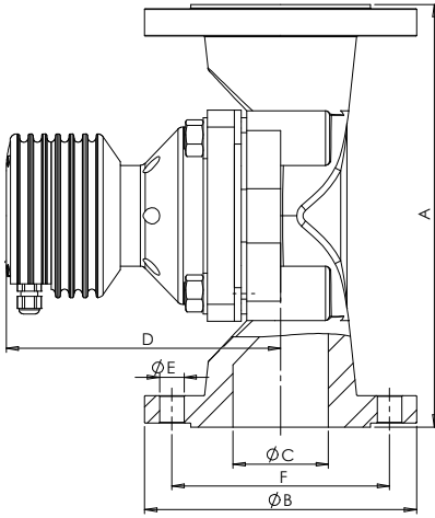
センサPR-23-W
