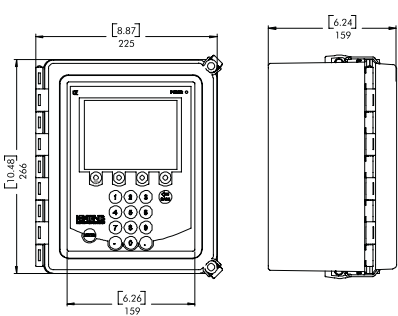
DTR変換器
