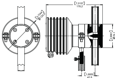
センサPR-23-M
