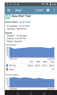
TCP or UDPフレーム iPerfスループットテスト
