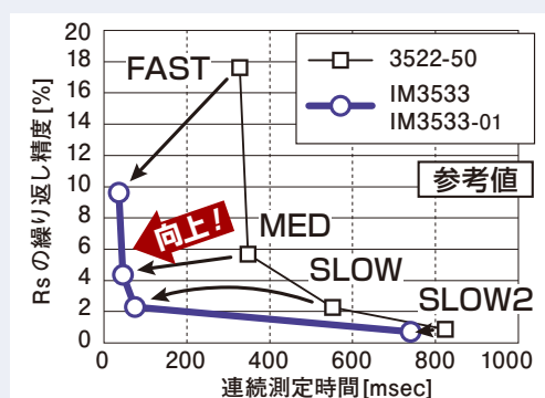
C-DとESR測定 (100 kHz) の連続測定時の 連続測定時間とRsの繰り返し精度 (サンプル: アルミ電解コンデンサ 1.5 \mu F)
