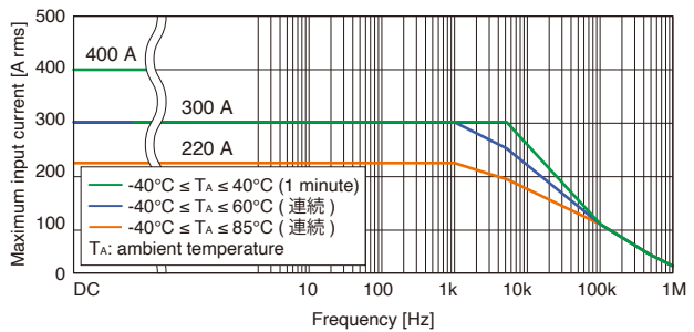
周波数特性 (代表特性例)
