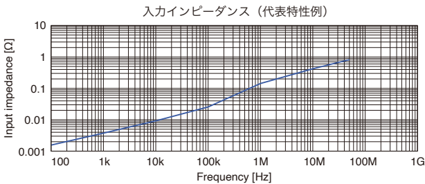
入力インピーダンス (代表特性例)
