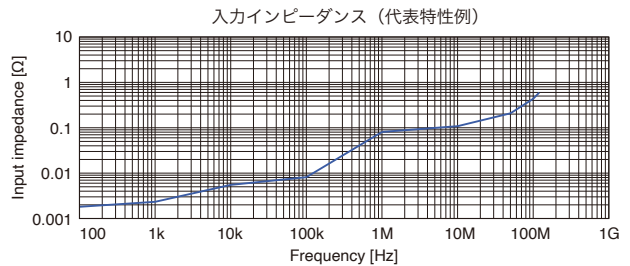
入力インピーダンス (代表特性例)
