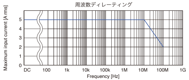
周波数ディレーティング
