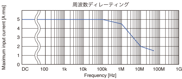
周波数ディレーティング
