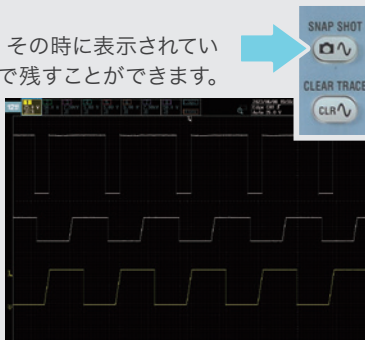
スナップショット使用例(白い波形)
