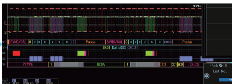
波形表示とデコード結果
