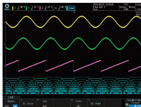
アナログ3チャンネル &amp; ロジック8bit
