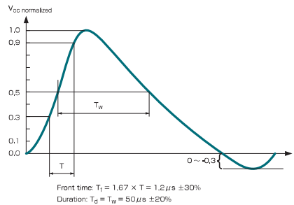
電圧波形
