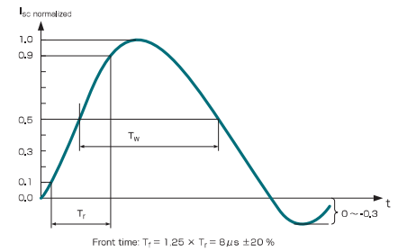
電流波形
