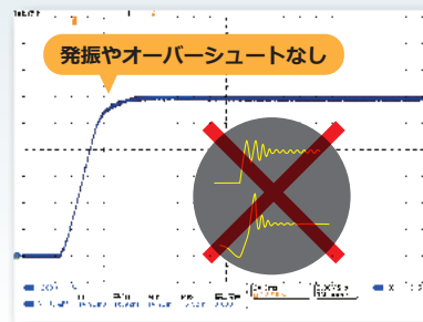
400 μF のコンデンサを接続した出力電圧波形
