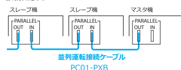
接続概念図
