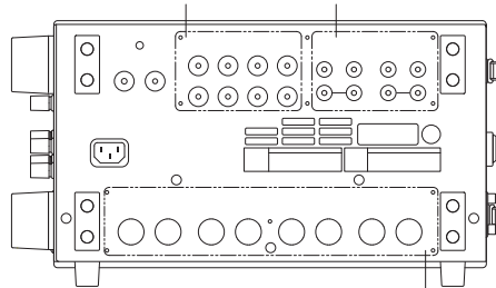
背面図(端子保護カバーなし)
